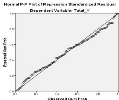
Gambar 2 Grafik Uji Normalitas Probability Plot dengan IBM SPSS Statistics 23
